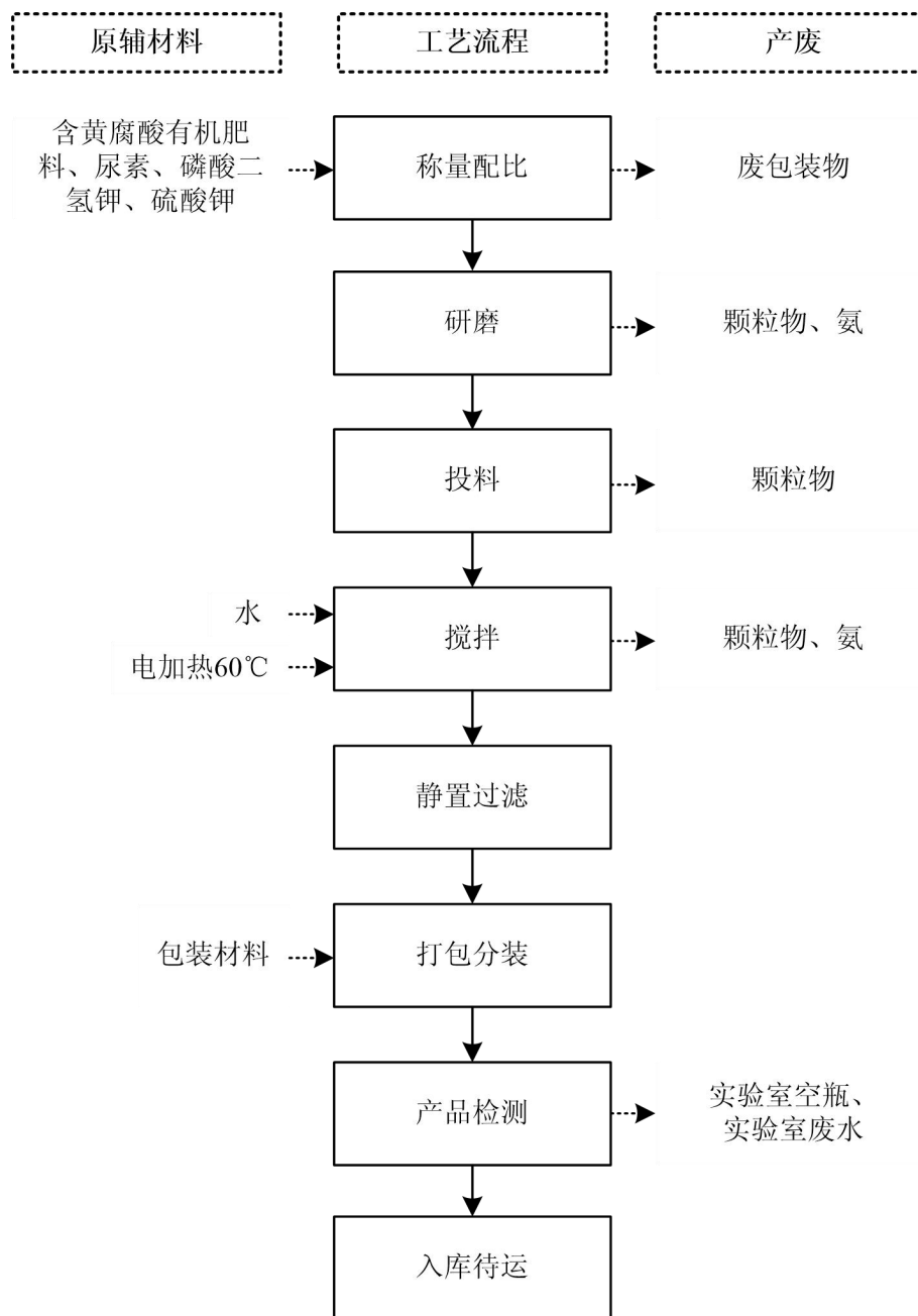
图 2-4 运营期生产工艺流程图
